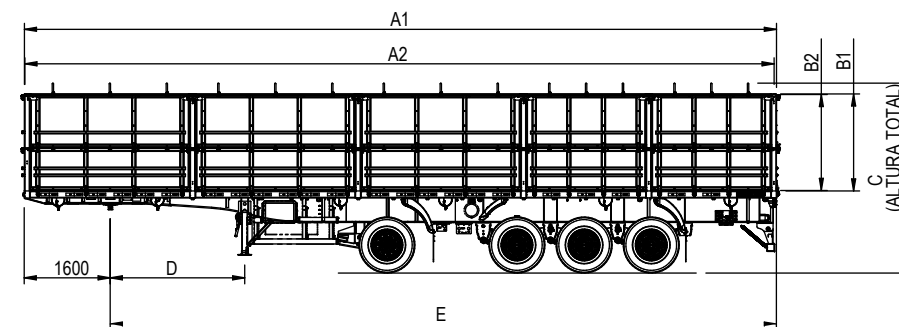
DESENHO TÉCNICO
