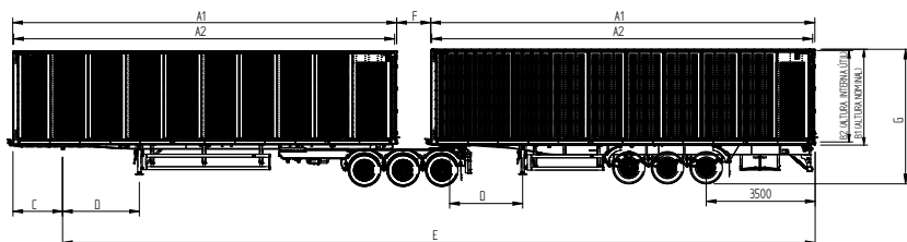
DESENHO TÉCNICO
