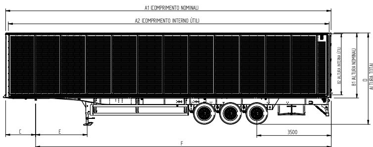
DESENHO TÉCNICO
