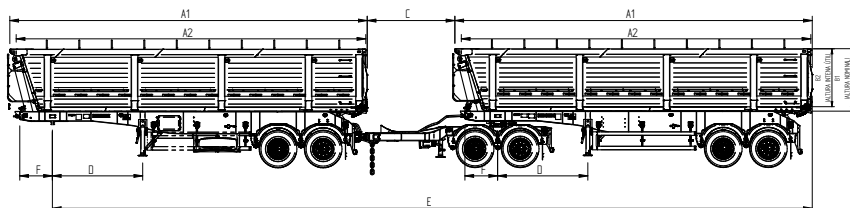
DESENHO TÉCNICO
