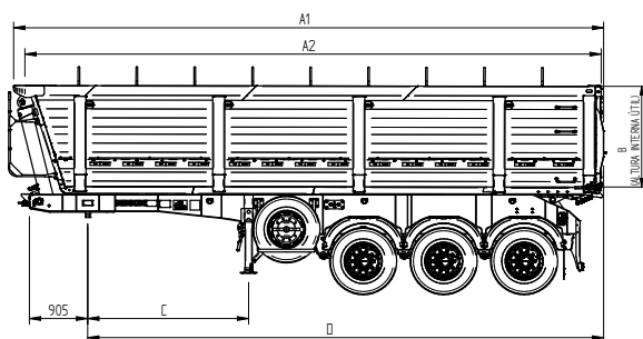
DESENHO TÉCNICO
